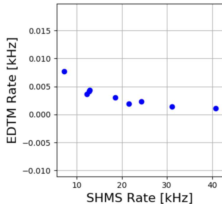
SHMS LH2 5342-5366
