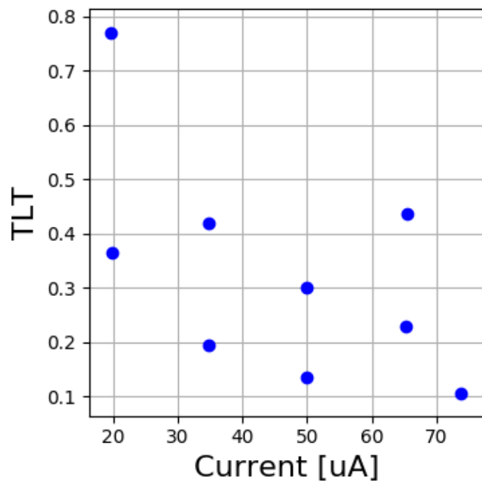
LH2 5342-5366
