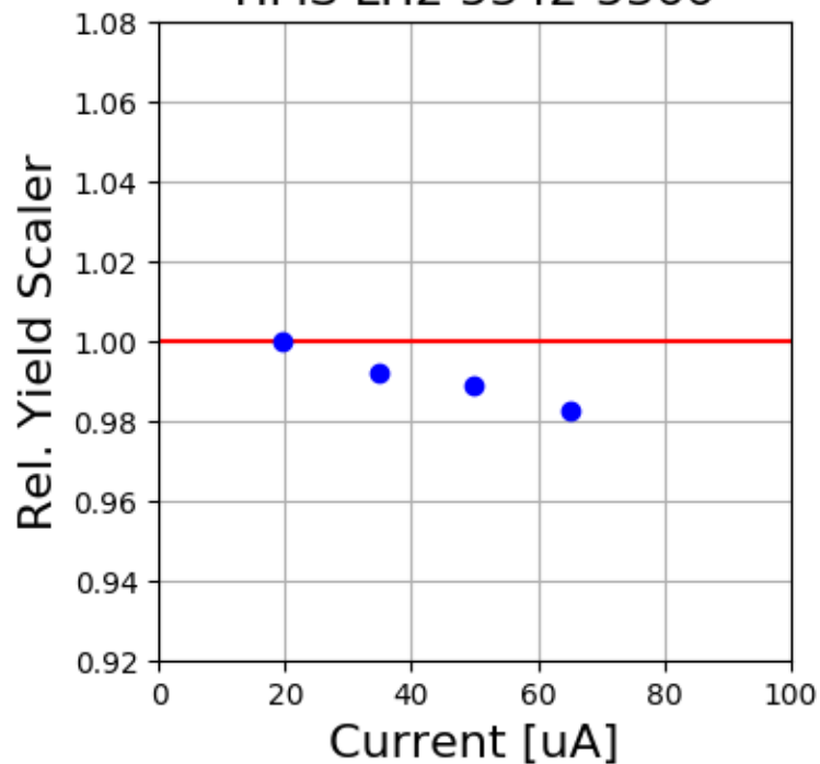
SHMS LH2 5342-5366
