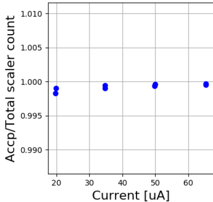
LH2 5342-5350
