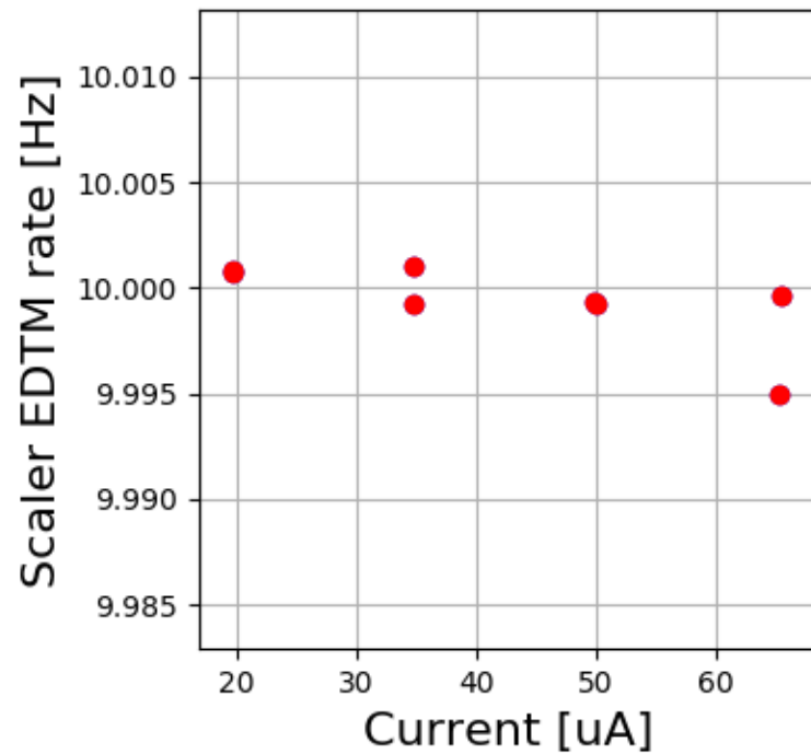
HMS LH2 5342-5350
