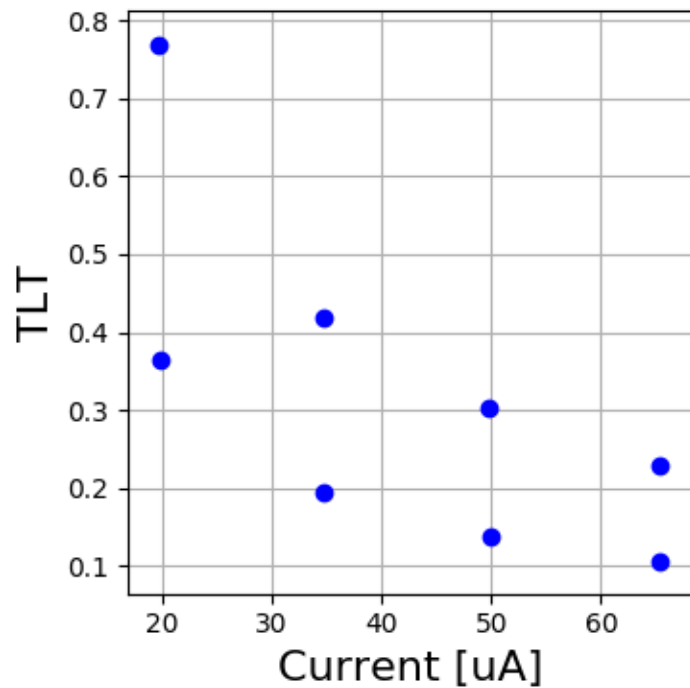
LH2 5342-5350
