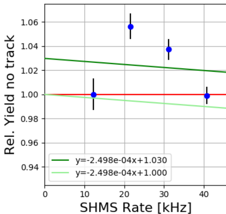
SHMS LH2 5342-5350
