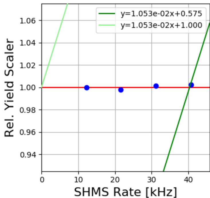
SHMS LH2 5342-5350
