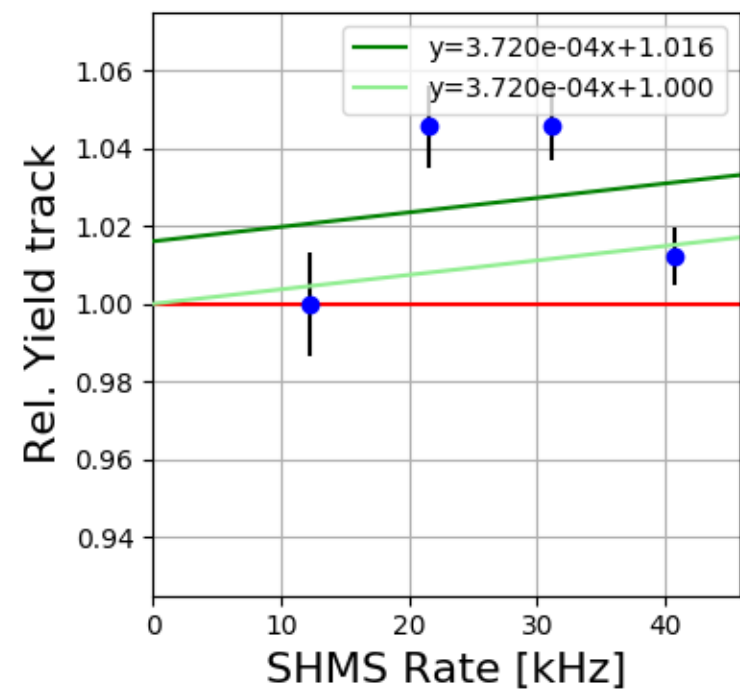
SHMS LH2 5342-5350
