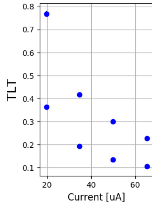
LH2 5342-5350
