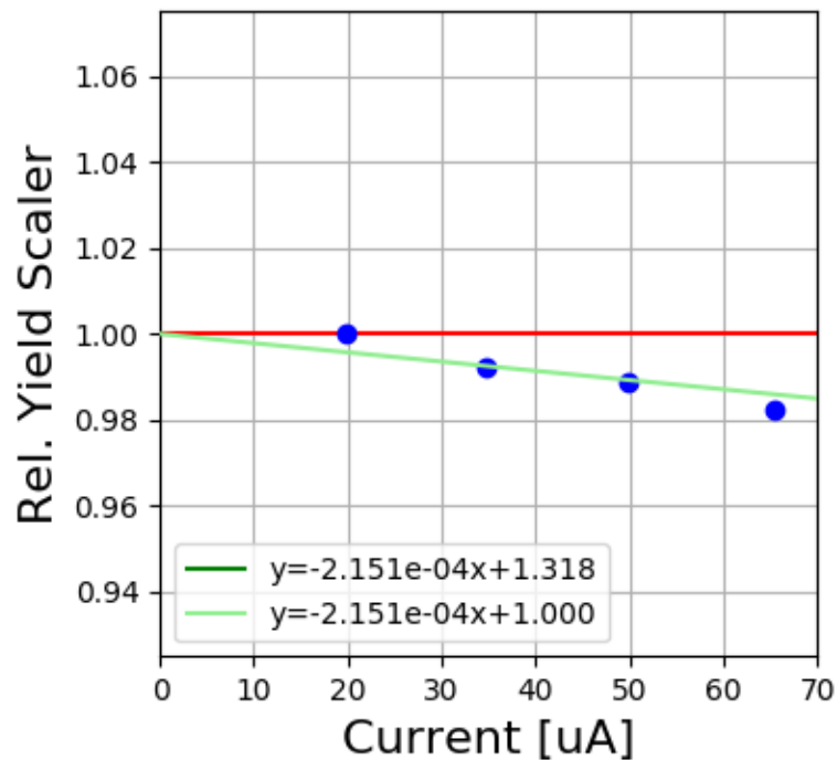
SHMS LH2 5342-5350
