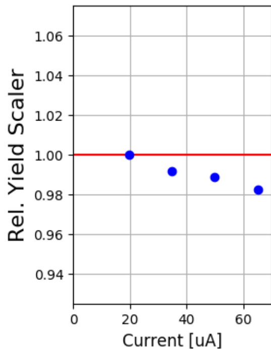
SHMS LH2 5342-5350
