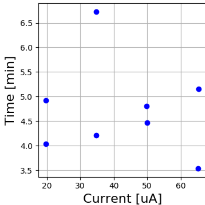
HMS LH2 5342-5350
