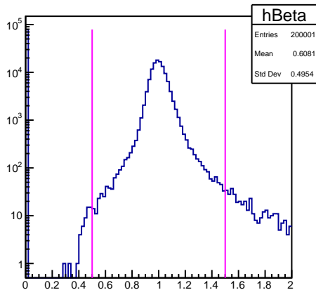
H.hod.beta
