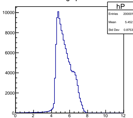
H.gtr.p
