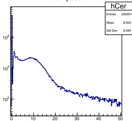
H.cer.npeSum
