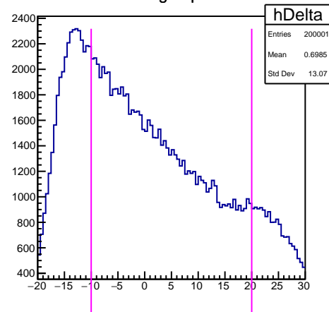
H.gtr.dp
