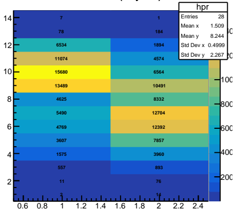
Preshower (Layer1)
