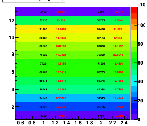
Preshower (Layer1)
