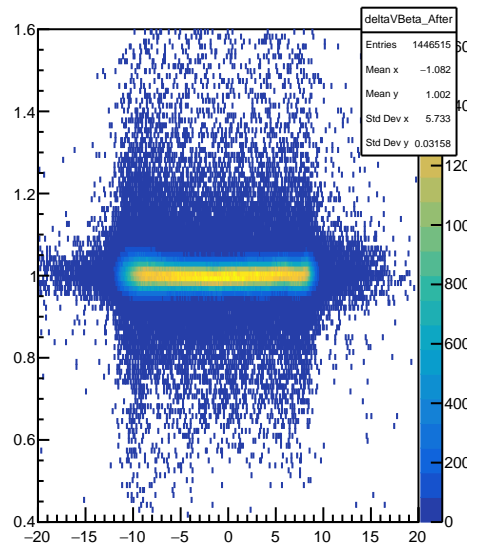
deltaVBeta_After
