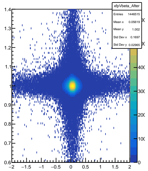
xpvbeta_After
