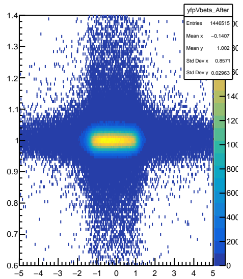
yfpvbeta_After
