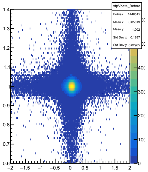
xpvbeta_Before
