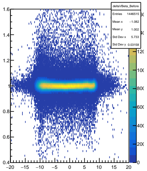
deltaVBeta_Before
