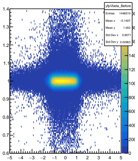
yfpvbeta_Before
