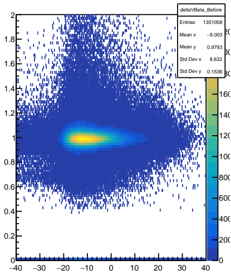
deltaVBeta_Before
