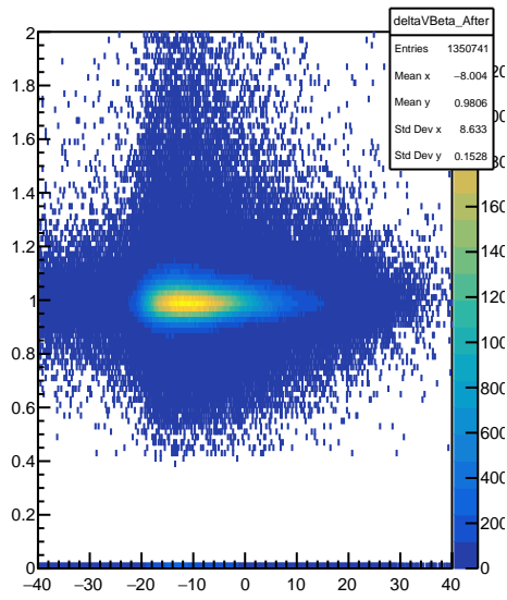
deltaVBeta_After
