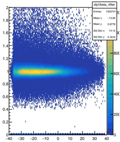
xpvbeta_After
