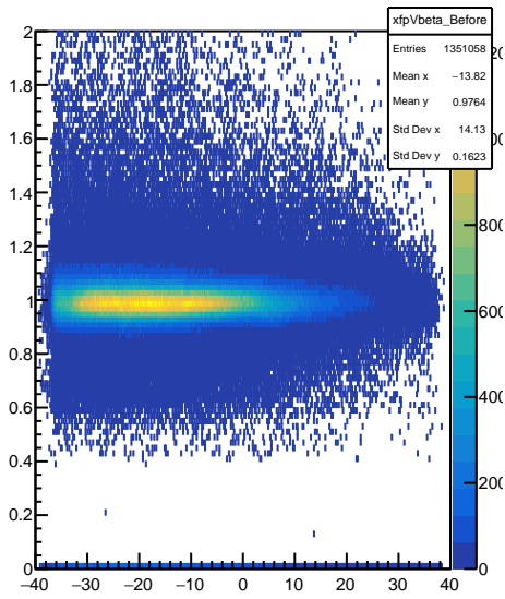
xpvbeta_Before
