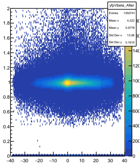
yppvbeta_After
