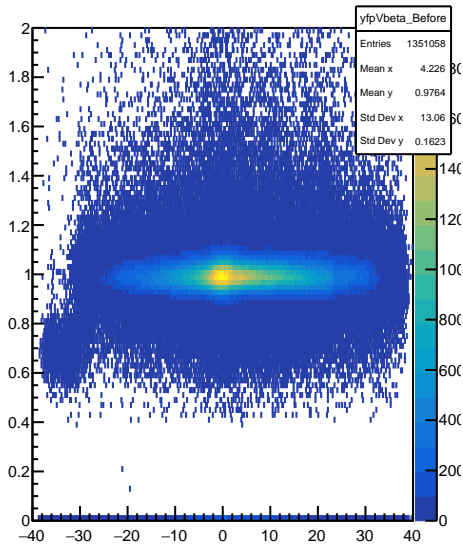
yppvbeta_Before
