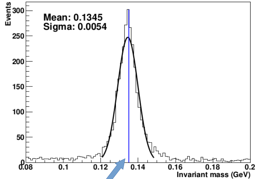
Invariant Mass (GeV)
