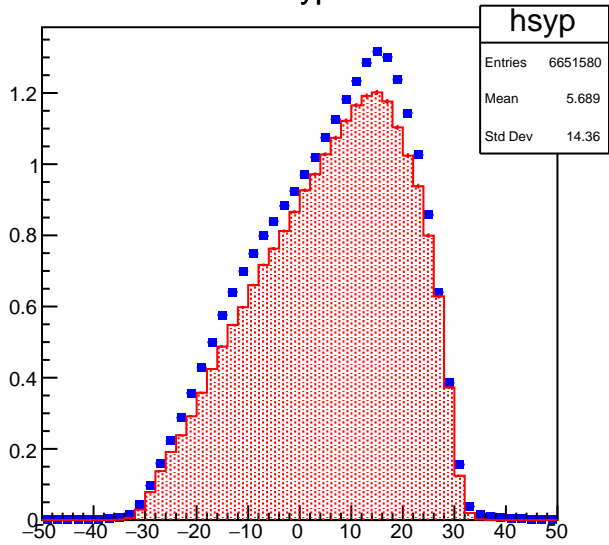
Data yptar
