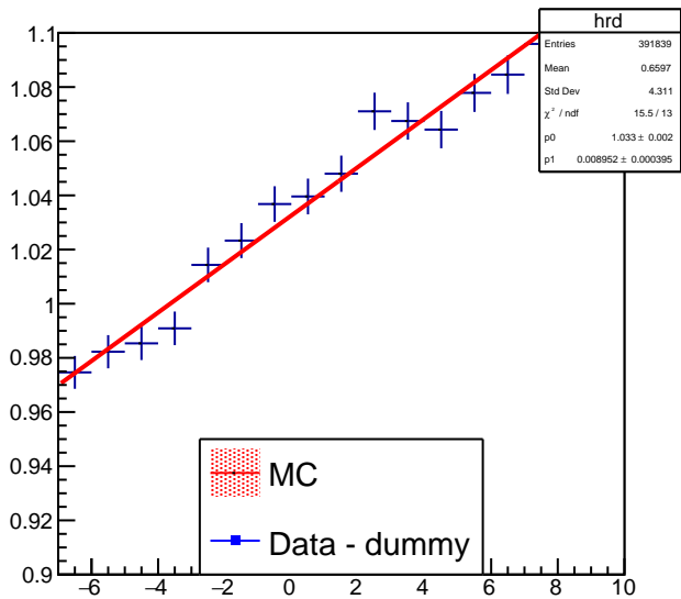
Ratio Data/MC
