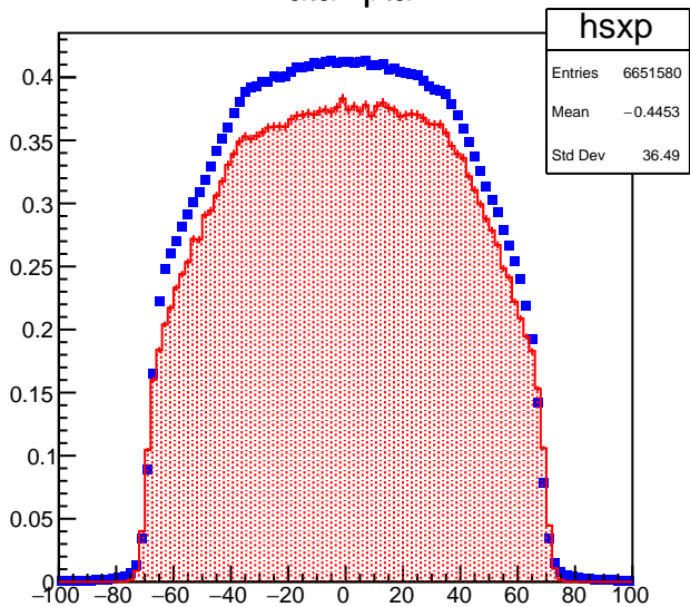
Data xptar
