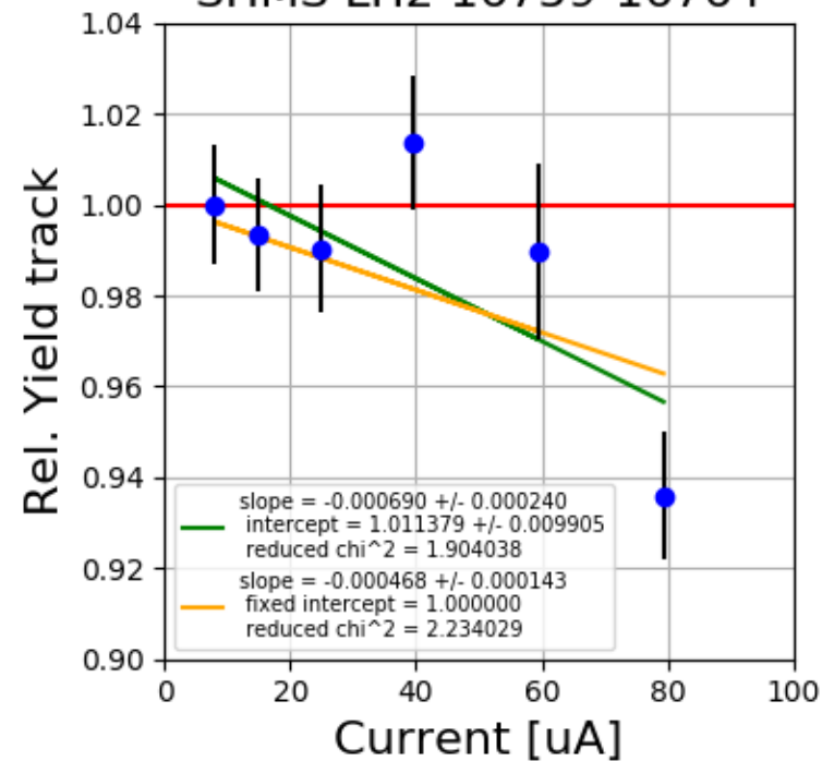
SHMS LH2 16759-16764
