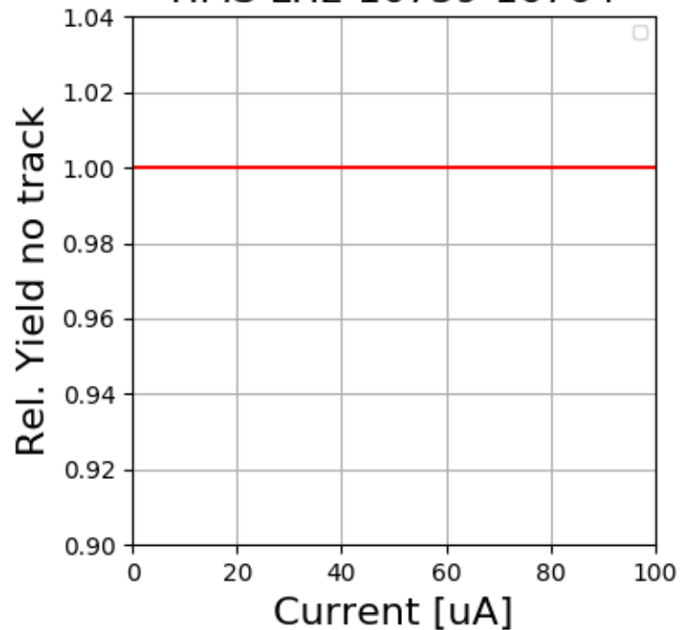
SHMS LH2 16759-16764
