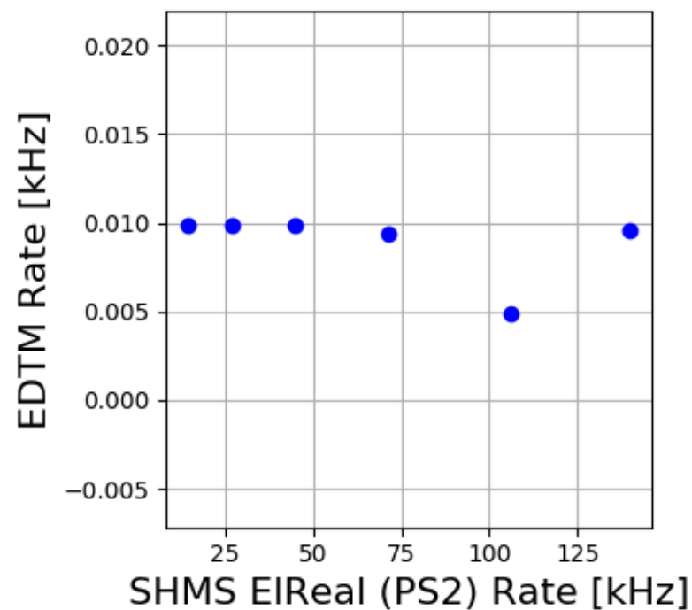
SHMS LH2 16759-16764
