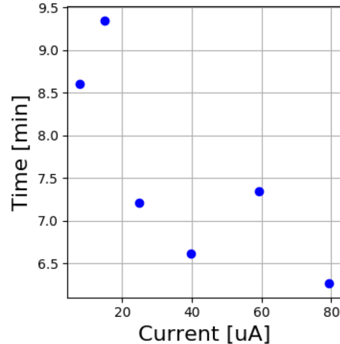
HMS LH2 16759-16764
