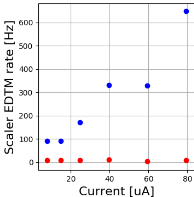
HMS LH2 16759-16764
