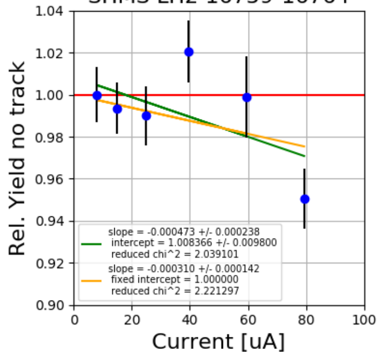
SHMS LH2 16759-16764
