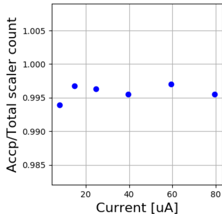
LH2 16759-16764
