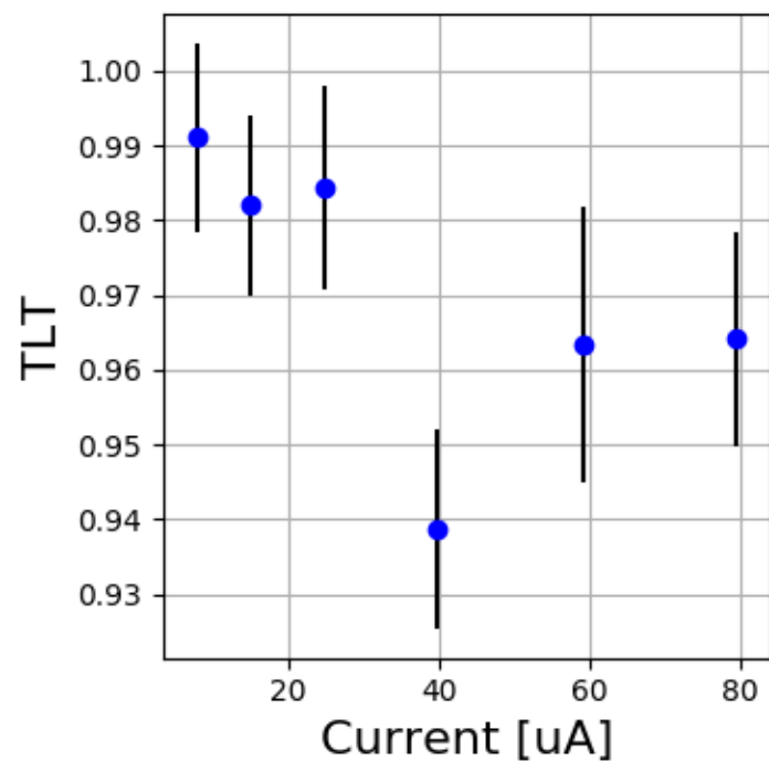
LH2 16759-16764
