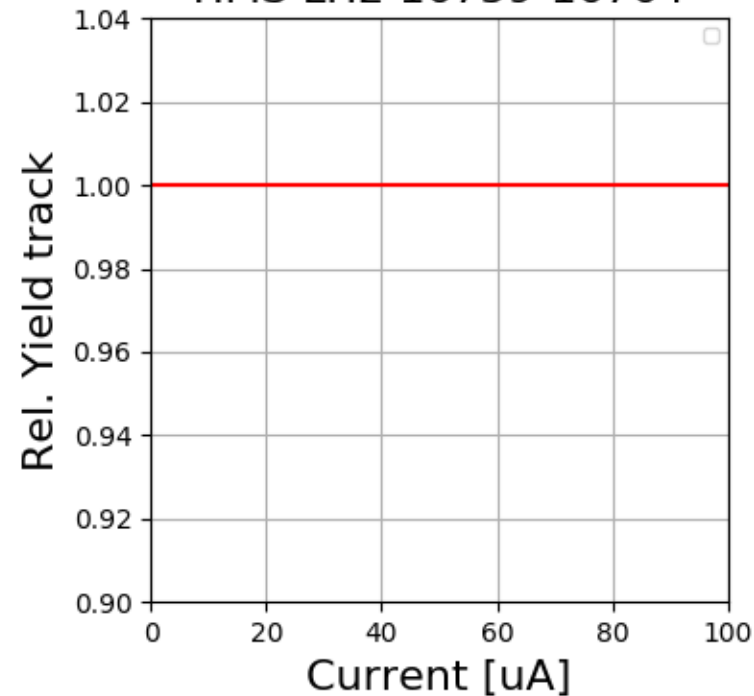
SHMS LH2 16759-16764
