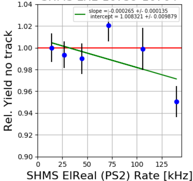
SHMS LH2 16759-16764
