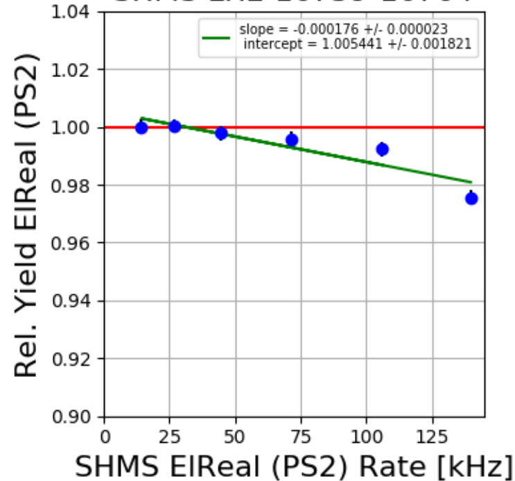
SHMS LH2 16759-16764
