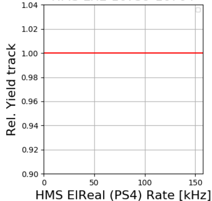
SHMS LH2 16759-16764
