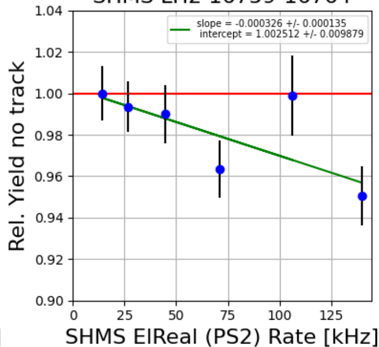
SHMS LH2 16759-16764
