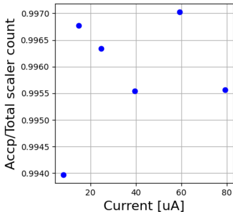
LH2 16759-16764
