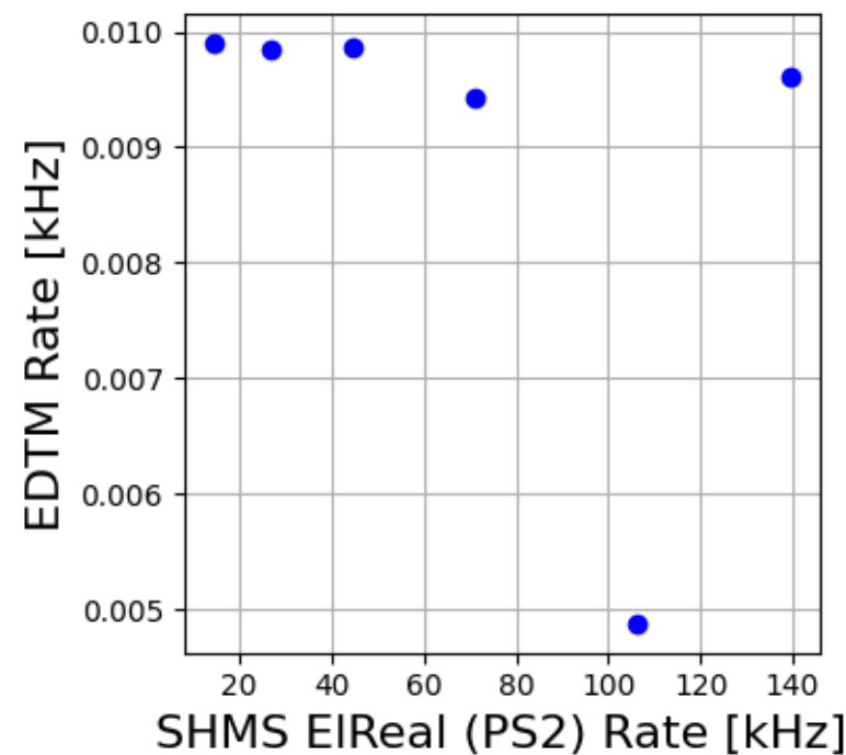
SHMS LH2 16759-16764
