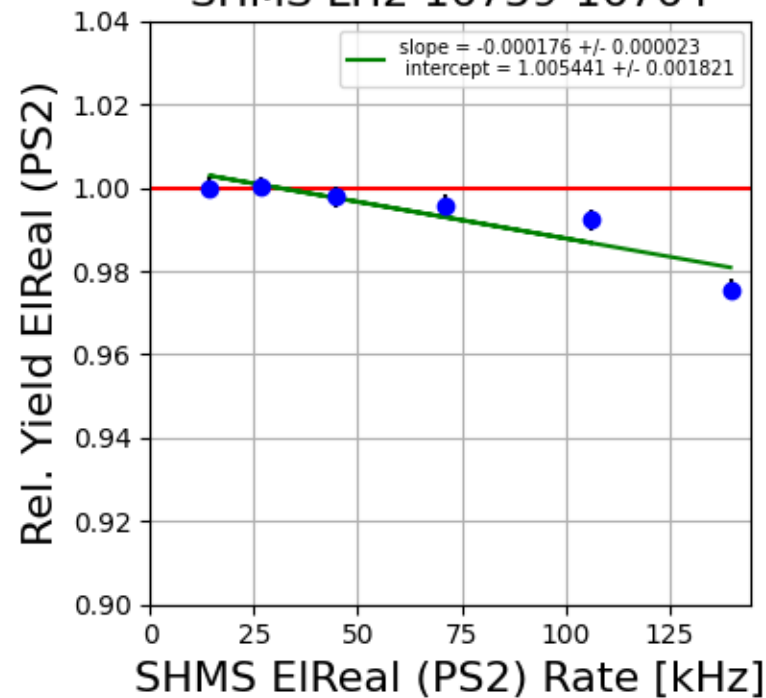
SHMS LH2 16759-16764
