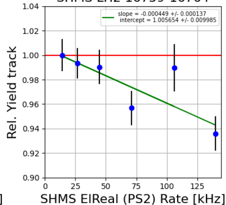
SHMS LH2 16759-16764
