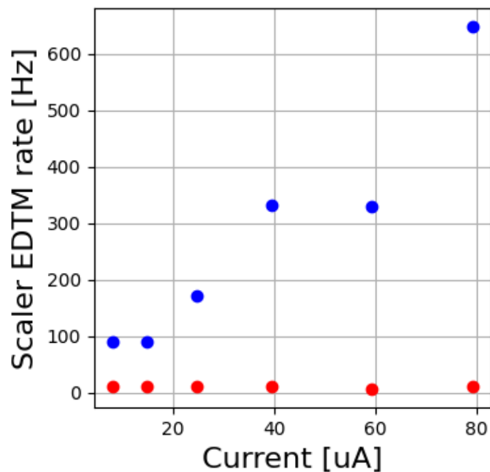
HMS LH2 16759-16764
