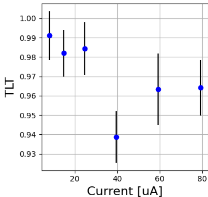
LH2 16759-16764
