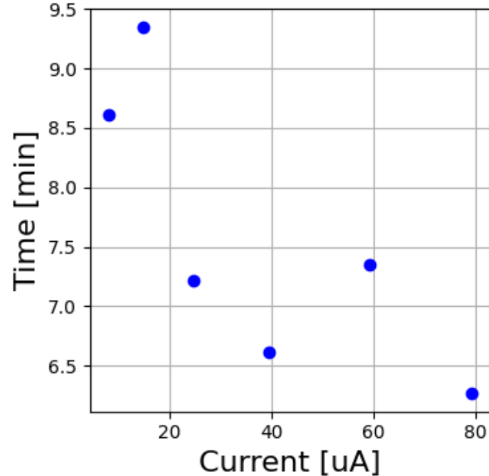
HMS LH2 16759-16764
