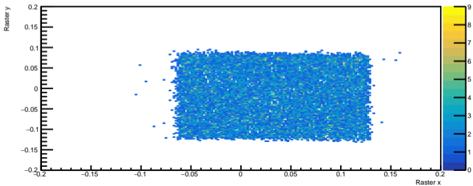
Raster x vs Raster y
