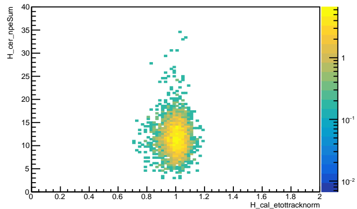
HMS cal etotracknorm vs HMS cer npeSum (random+acpt_cut)
