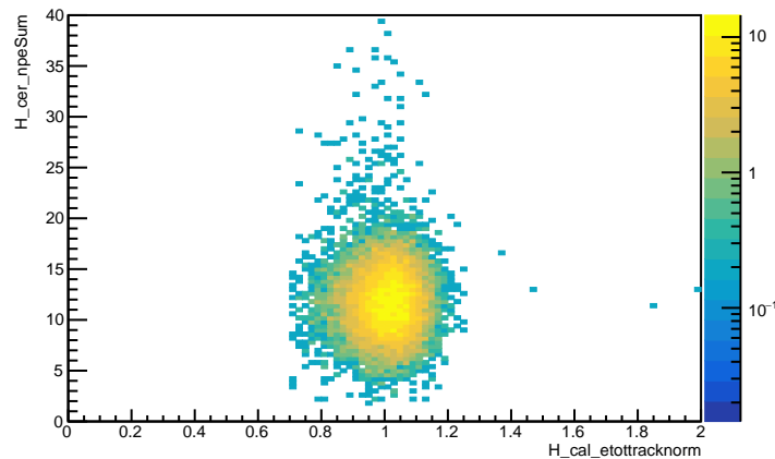
HMS cal etotracknorm vs HMS cer npeSum (random+accpt_cut)
