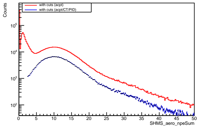
SHMS aero npeSum (accpt_cut)
