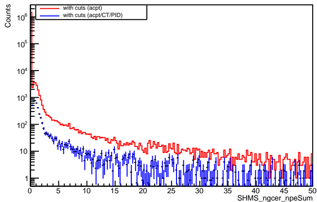
SHMS NGC npeSum (accpt_cut)
