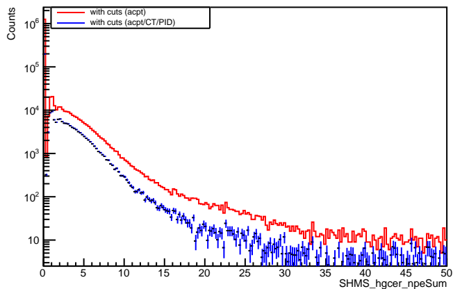
SHMS HGC npeSum (accpt_cut)
