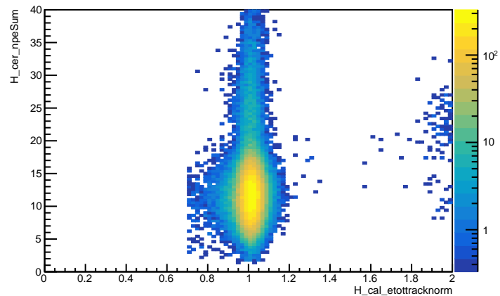
HMS cal etottracknorm vs HMS cer npeSum (random+acpt_cut)
