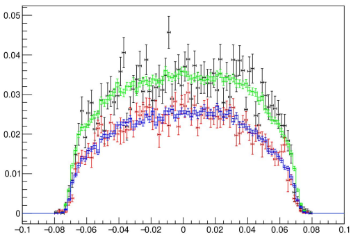
HMS xptar
