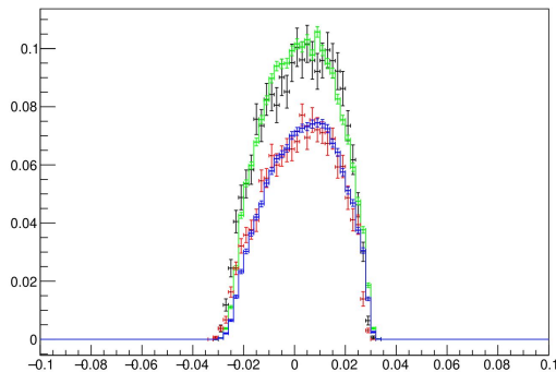
HMS yptar
