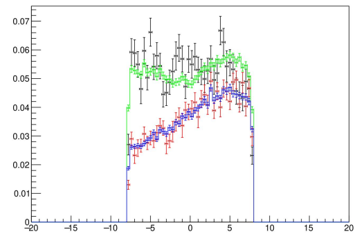
HMS Delta
