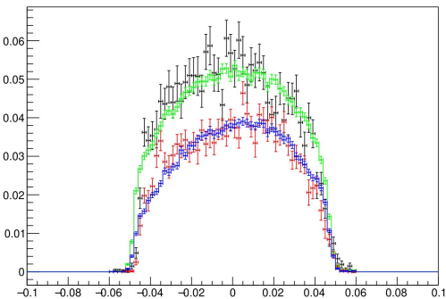
SHMS xptar
